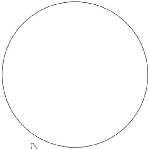
Júpiter
