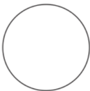
Netuno
