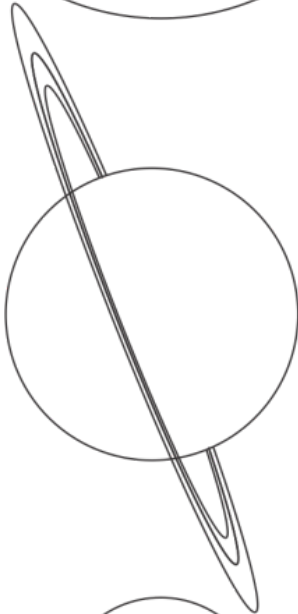
Urano
